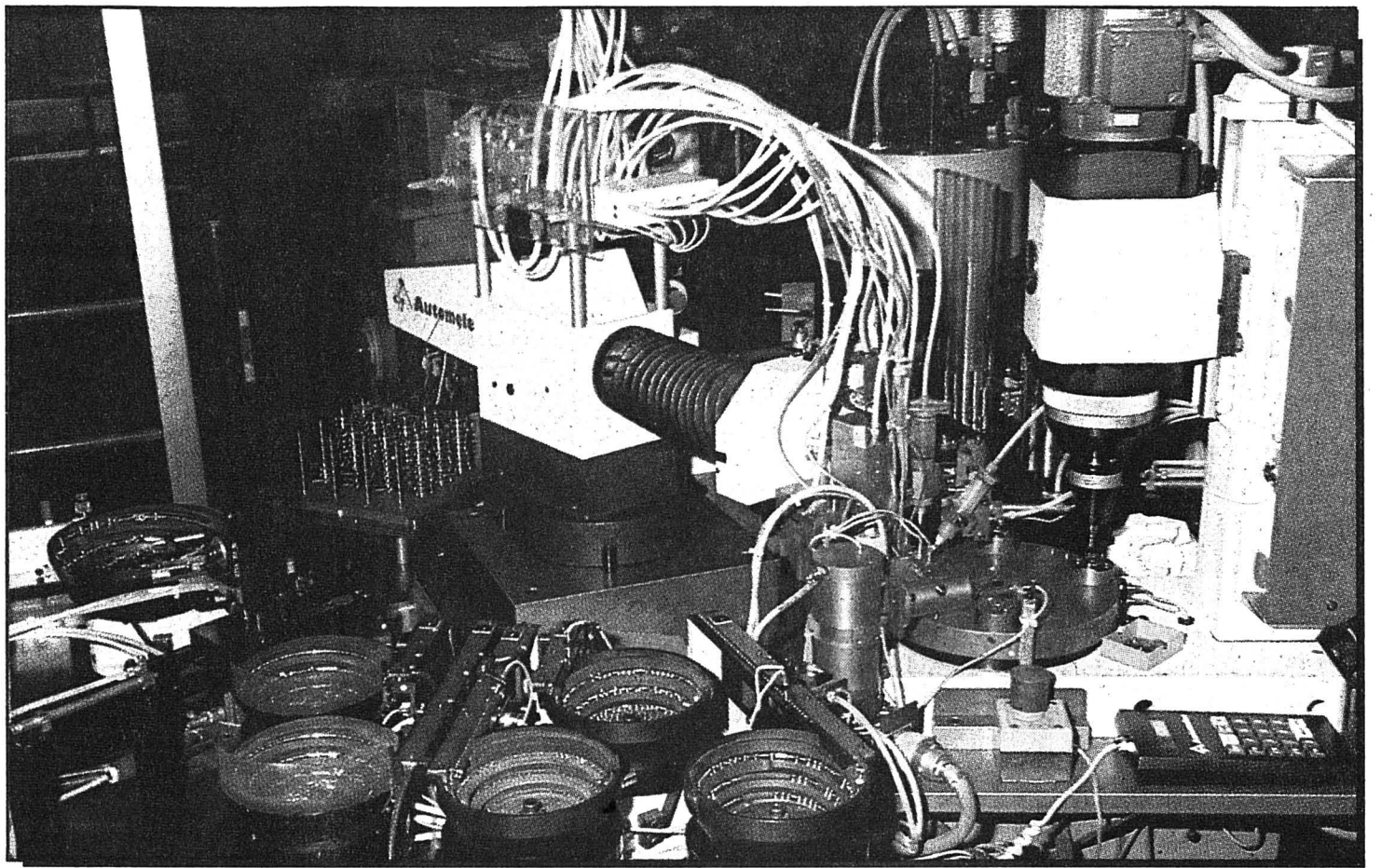
Un robot de Automelec, à Tramelan. Les chercheurs travaillent à une nouvelle génération: des robots autonomes qui n'auront plus besoin d'un lien ombilical avec un ordinateur central, mais capables de générer leur propre programme... (Photo Impar-Gerber)
