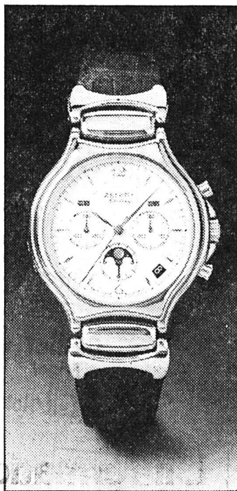
Le chronographe «Academy» de Zenith, parfait exemple de la montre «compliquée» très en vogue aujourd'hui. Mouvement automatique à fréquence élevée (36.000 Ah), rotor central sur roulement à billes, réserve de marche min. 50 heures. Mesure le 1/10e de seconde, avec petite seconde et totalisateurs de minutes et d'heures. Calendrier instantané, jour - mois - phases de lune. (Zenith «Academy»)
