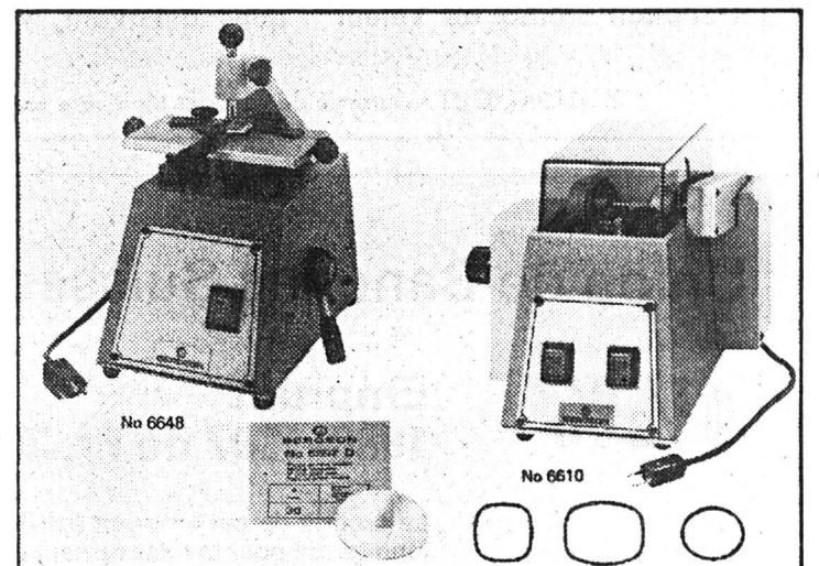
Les branches annexes de l'horlogerie occupent une place importante dans les salles de la FEHB. La maison Bergeon & Cie au Locle est fidèle au rendez-vous avec ici une machine à façonner les empreintes pour meuler les verres minéraux, ainsi qu'une machine automatique à meuler les verres minéraux de forme.
