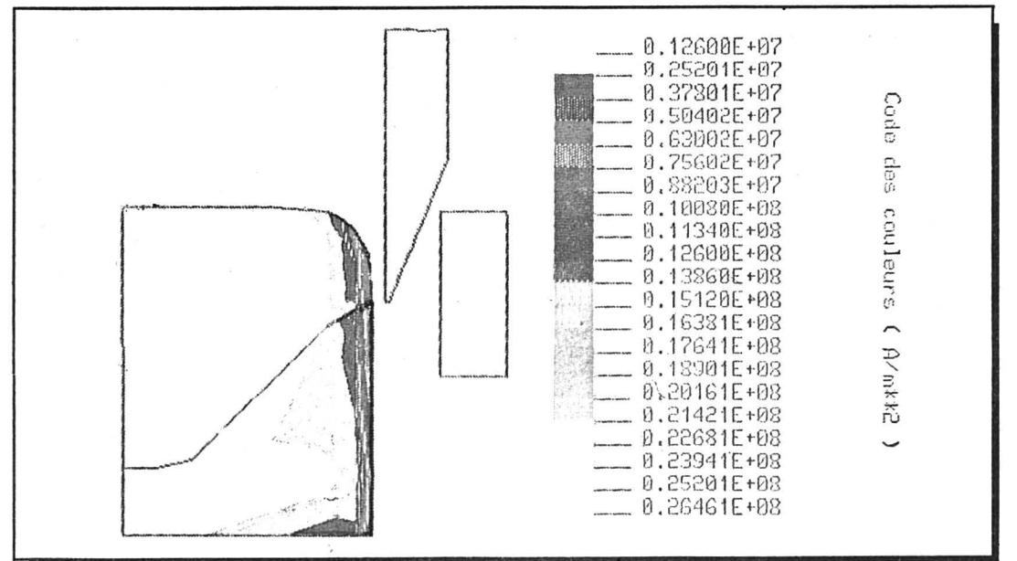
Densité du courant efficace dans une demi-section verticale du lingot calculée par le groupe Université de Neuchâtel et EPFL. L'effet pelliculaire y est nettement visible. Figure 3.
