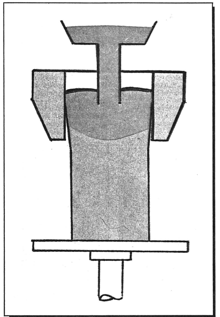
Schéma du procédé classique d'un métal (avec lingotière): métal liquide (bleu), métal solidifié (vert), lingotière (brun). Figure 1
