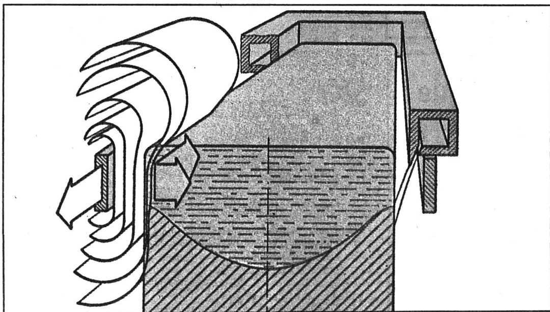
Schéma du procédé de coulée électromagnétique d'un métal: métal liquide (bleu), métal solidifié (vert), inducteur (brun). Les surfaces entourant l'inducteur correspondent à des valeurs constantes du champ d'induction magnétique. Les flèches situées dans le métal indiquent la direction des forces. Figure 2.
