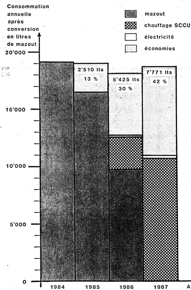
Les économies d'énergie sur le bâtiment Serre 14: 42% en équivalence mazout après raccordement au chauffage à distance et installation d'une pompe à chaleur. (Dessin M. Grünig)
