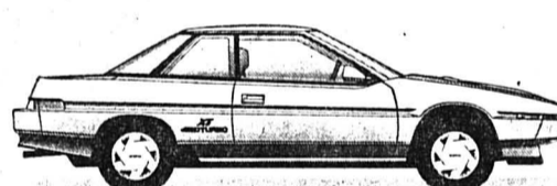
Subaru 1.8 XT Turbo 4WD , traction permanente 4x4 à différentiel central, 5 vitesses, 120 CV DIN, servo-direction, suspension indépendante électropneumatique à compensation automatique de niveau et réglage en hauteur, Fr. 32 200.-.
