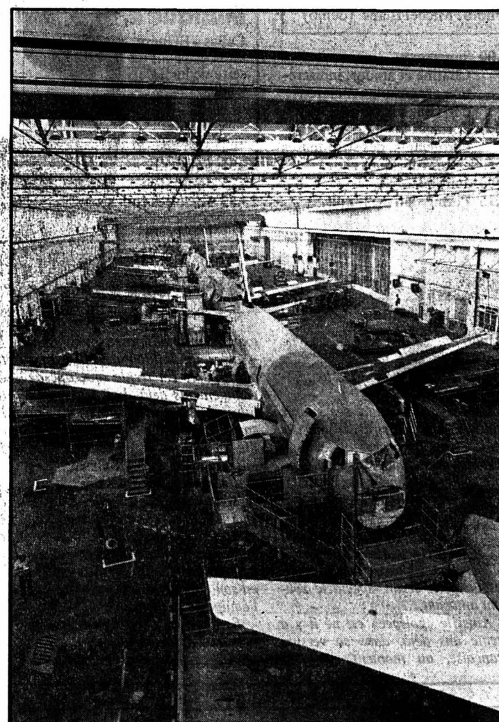
Airbus Industrie à Toulouse: la chaîne d'assemblage finale de l'A320. (photos Airbus Industrie).
