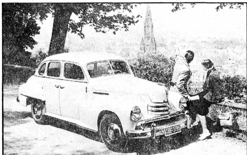
«Kapitän» 1951 - la grande Opel. La «Kapitän» fut considérée comme l'une des voitures les plus rapides et les plus luxueuses des années 50. Son moteur six cylindres développait 58 ch à 3700 tours/minute. Vitesse de pointe: 128 km/h.
