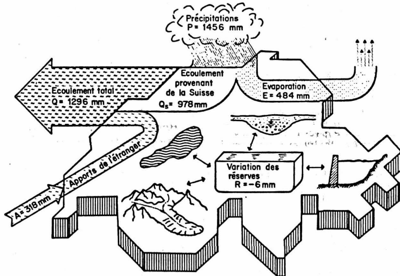
Bilan hydrique de la Suisse, de 1901 à 1980. 1456 mètres de précipitations en moyenne annuelle. (off. féd. de la protection de l'environnement).
