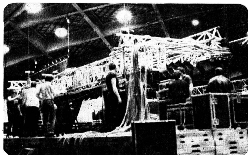
Avant de monter le pont d'éclairage, les branchements et vérifications sont effectués avec soin. (photos dn)
