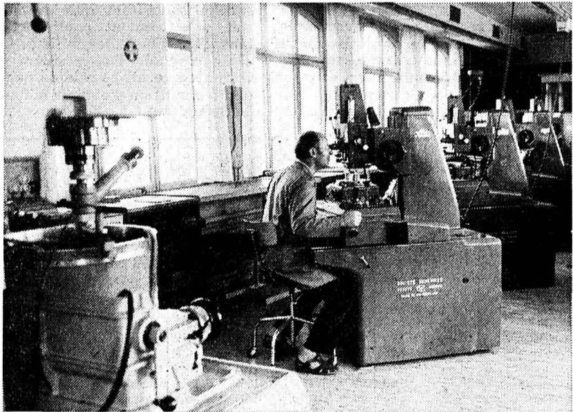
Le cadran à l'instar des autres composants de la montre, est une œuvre de précision. Ici le travail sur la machine à pointer pour la réalisation des étampes.
