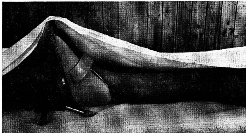
Le Paradolor, tel qu'il se présentait en cours de réalisation. Manque la gouttière. La base a été développée de manière à permettre de régler l'inclinaison du pied. La photo montre comment l'appareil supporte le poids du drap. Le pied est surélevé, soulageant le mollet.
