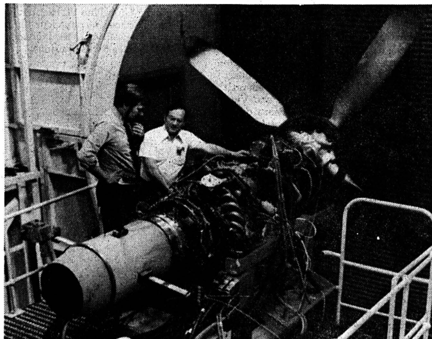
Le turbopropulseur Pratt & Whitney PW-100 à technologie avancée fabriqué au Canada et qui va équiper de nombreux avions de transports régionaux de 30 à 40 places.
