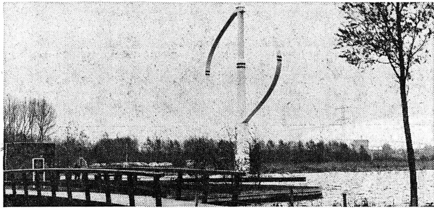
L'éolienne type Darrieus: simple, robuste, relativement silencieuse et non dépourvue d'élégance. Ces sortes d'«oignons» pourraient remplacer, au pays des tulipes et ailleurs, les moulins à vent classiques. (photo BBC)
