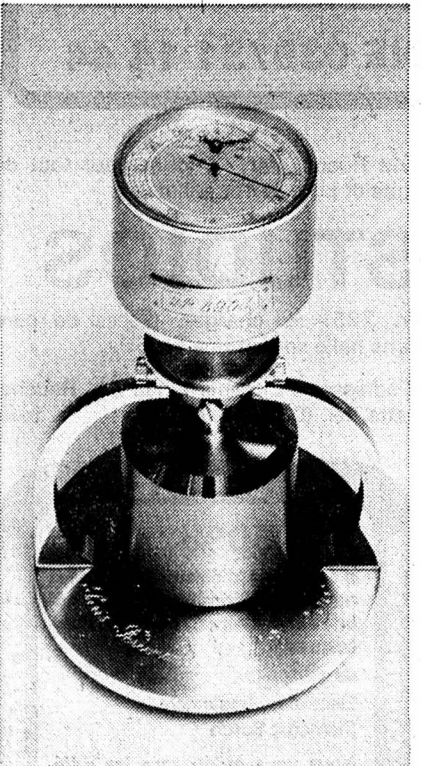
Reproduction d'un chronomètre de marine - pièce unique - réalisée par le maître horloger suisse Ferdinand Berthoud en 1796. Cadran à heures et minutes décentrées. Seconde au centre. Boîtier acier et laiton polis. Reproduction de la suspension à cadran originale, avec contrepoids. Equipé d'un mouvement Imhof à quartz (4 MHz) muni d'un certificat du Contrôle officiel des chronomètres COSC. L'original fait partie des collections du Musée international d'horlogerie à La Chaux-de-Fonds. Une pièce signée Imhof, La Chaux-de-Fonds.
