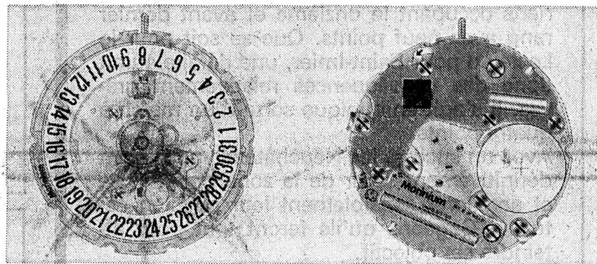
Calibre ESA 10 1/2 928.411, quartz seconde au centre, quantième instantané correcteur, dispositif stop, de la famille ESA QUARTZ II, exécuté en «Marinium».
