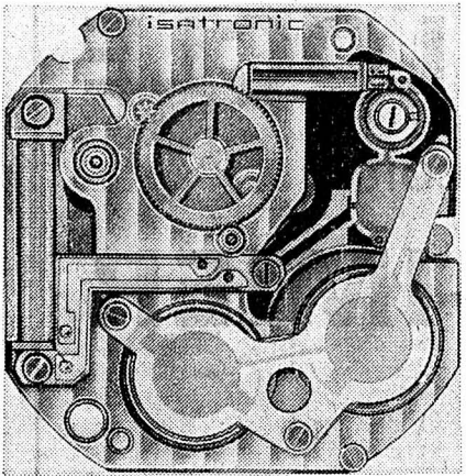
La pile au lithium à large autonomie est apparue: un peu de technique avec ce représentant de la famille de mouvements Isatronix, La Chaux-de-Fonds (groupe Voumard) toutes les parties mobiles, moteur compris, sont montées sur roulements à billes assurant ainsi une résistance à toute épreuve aux chocs et à l'usure. Il s'agit de 6/8 lignes hauteur 1,60 mm, pile comprise 9 lignes 1,60 mm, pile comprise également et d'un 10 1/2 lignes hauteur 1,20 mm, avec pile au lithium de 12 ans d'autonomie ou pile classique.
