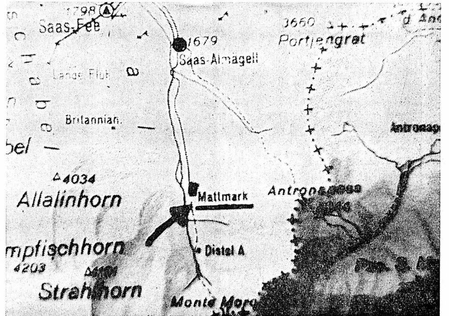
La flèche indique le mouvement de l'éboulement à Mattmark, entre Saas-Almagell et le Monte-Moro.
