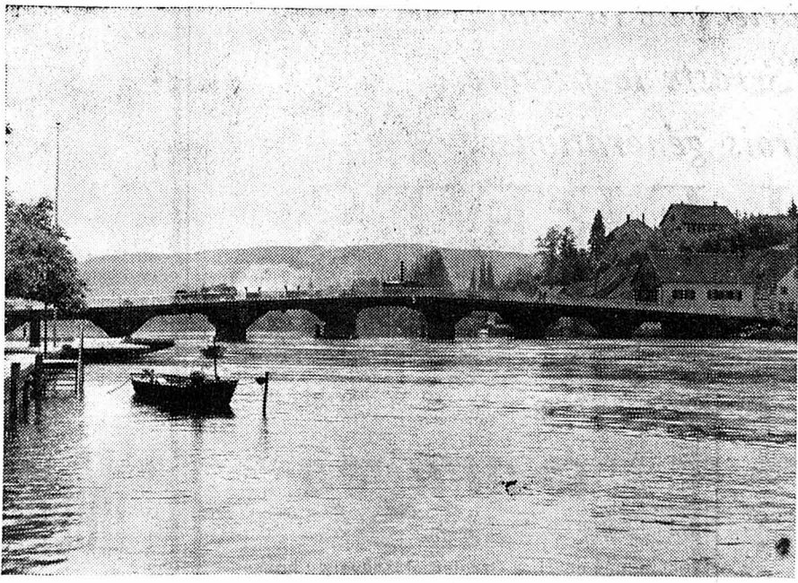
En six mois de travail, le pont sur le Rhin, à Stein am Rhein, a été remis en état. La chaussée a été portée de 4,95 à 6 mètres et les trottoirs des deux côtés, élargis de 80 centimètres, mesurent maintenant 2 mètres. Le pont a été renforcé et supporte 13 tonnes au lieu de 10 auparavant. Coût 350.000 frs. Notre photo montre le pont du Rhin dont la silhouette s'harmonise heureusement avec le paysage et les vieilles maisons de Stein am Rhein.
