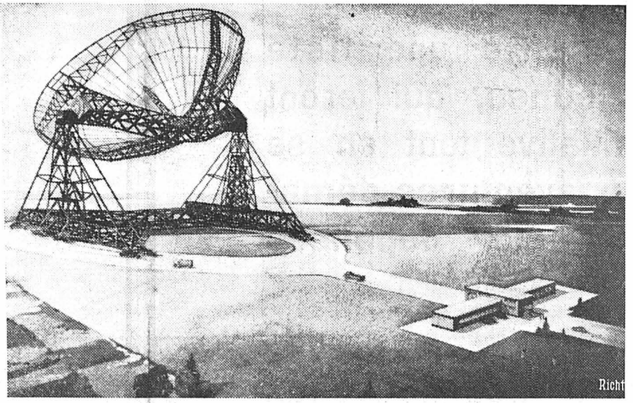
Un des problèmes que l'astronomie se propose de résoudre est celui des étoiles-radios qu'on ne peut observer au télescope mais qu'on mesure au moyen d'antennes spéciales. Pour mieux étudier ces étranges étoiles, une antenne-radar géante sera construite à la station d'essais de Jordell Bank (U. S. A.). Cette antenne, qui peut se mouvoir dans toutes les directions, aura un diamètre de 80 mètres.
