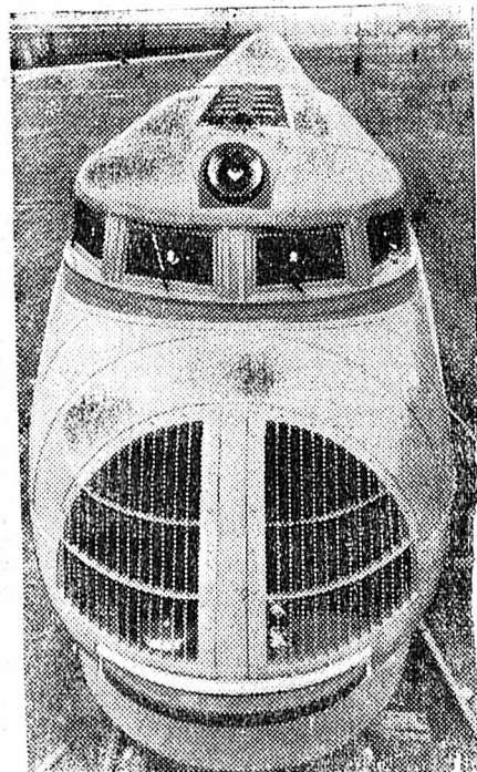
Cette machine, destinée à l'Union Pacific Railway, est munie d'un moteur de 600 C. V. et peut entraîner un convoi à une vitesse maximum de 160 km. à l'heure. — Le train entier ne pèse pas plus qu'un seul wagon de Pullman.
