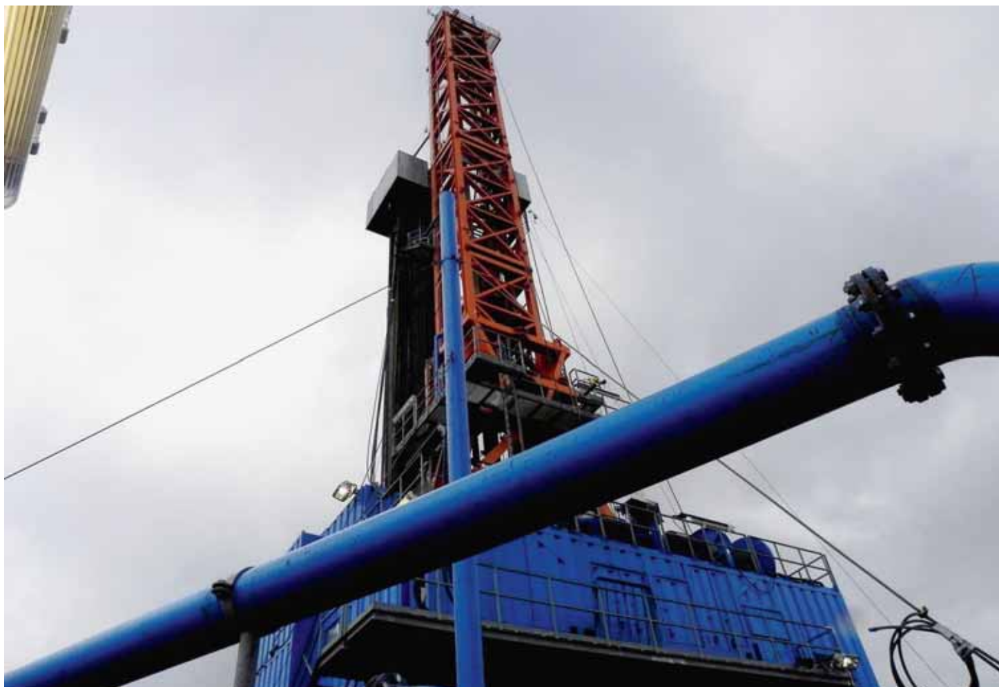
La tour du forage de Taufkirchen, à dix kilomètres de Munich, s'élève à près de cinquante mètres du sol.
