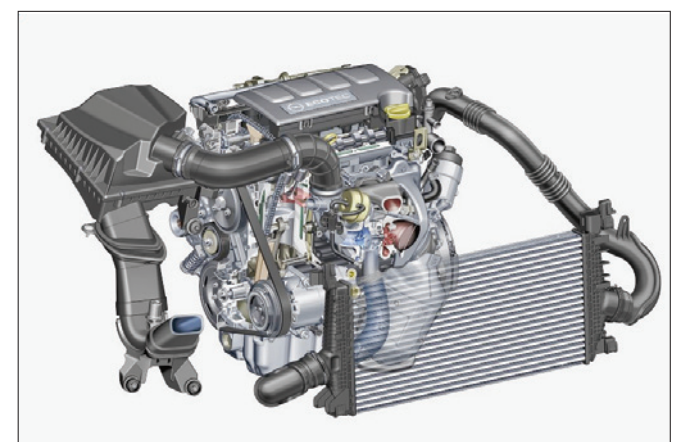
SMALL IS BEAUTIFUL Sur l'Opel Astra, ce moteur 1,4 litre turbo de 140 ch a remplacé le 1,8 litre atmosphérique de même puissance. Du coup, la consommation moyenne a chuté de 7,2 à 5,9 l/100 km (-18 %). (SP)
