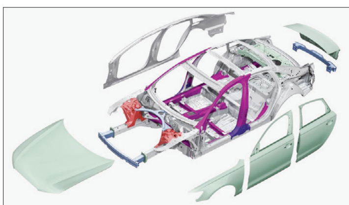
L'ENNEMI, C'EST LE POIDS Un recours accru à l'aluminium (notamment les panneaux vert pâle) et à des aciers à haute et très haute résistance a permis d'alléger la carrosserie brute de l'Audi A6 de 15%. (SP)
