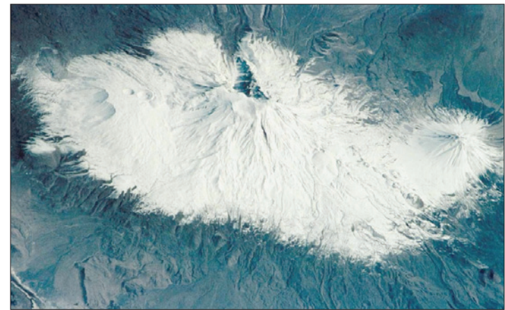
TURQUIE En utilisant des images satellites comme celle-ci, les scientifiques ont découvert que les glaciers du mont Ararat avaient perdu 30% de leur surface entre 1976 et 2008. (SP-NASA)
