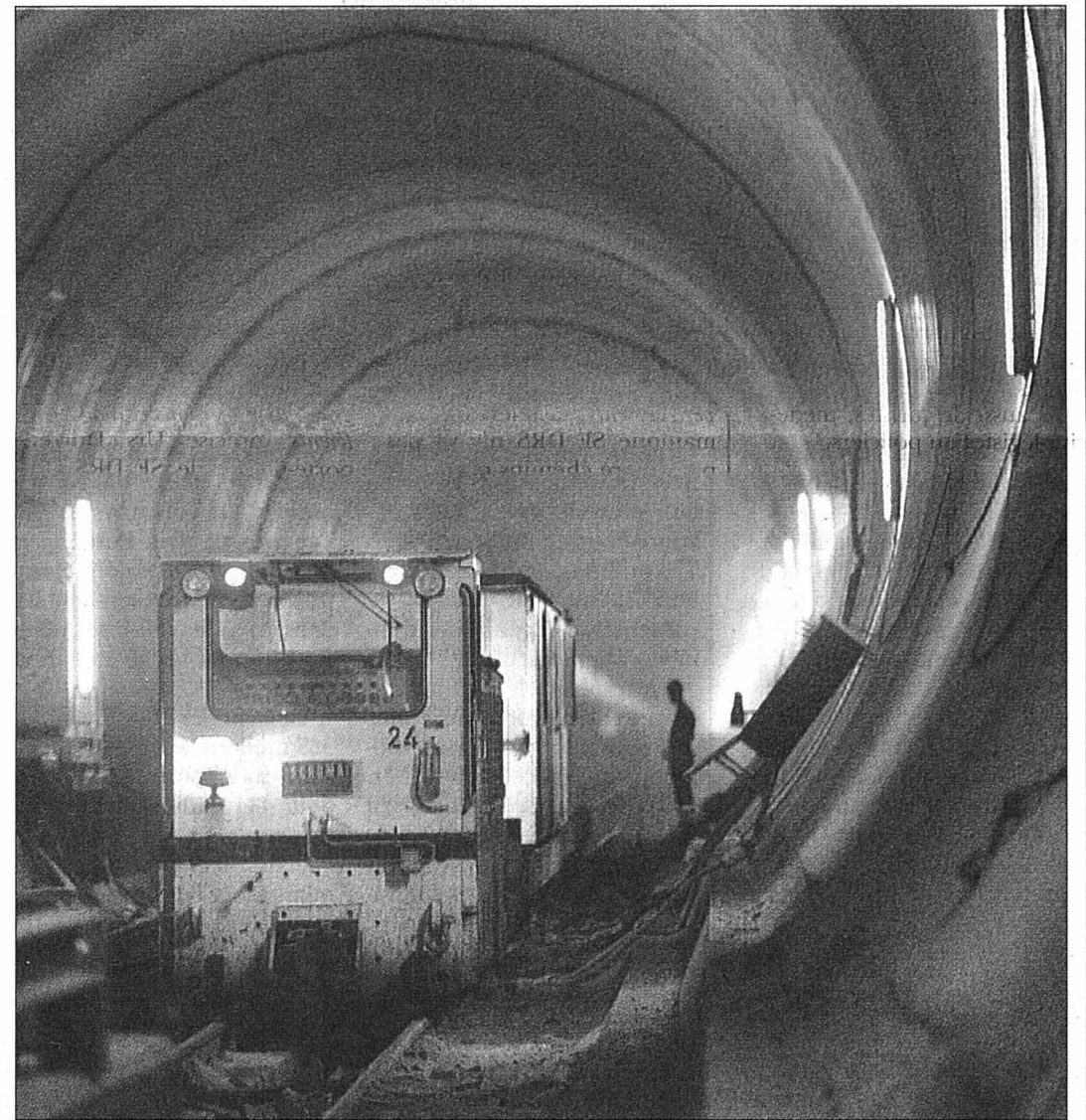
L'anneau intérieur du tunnel doit être bétonné sur toute la longueur. C'est quand tout cela sera achevé que pourra commencer l'équipement ferroviaire proprement dit. Il est prévu de poser 57 km de voies ferrées. PHOTO KEYSTONE
