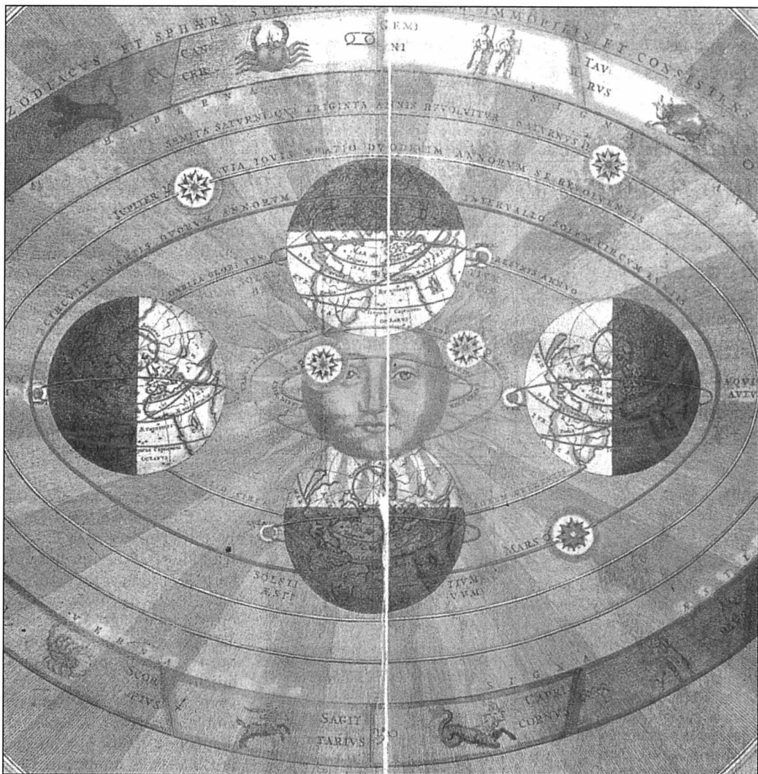
La surface terrestre a reçu de moins en moins d'énergie lumineuse ces dernières décennies. Le Soleil est hors de cause. La pollution et/ou un surcroît de nuages dû au réchauffement filtreraient la lumière visible et l'infrarouge. Les UV, eux, passent toujours en excès, à cause d'une couche d'ozone effilochée...
