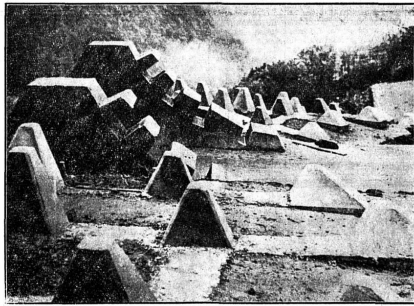
Un des aspects du dispositif de défense de la ligne Siegfried
