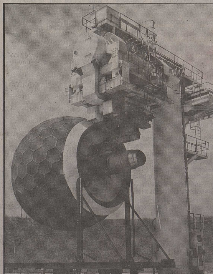
Etrange balle de golf? Non, un banc d'essai pour réacteurs à Hucknall, près de Nottingham.
