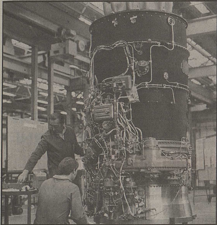
Un moteur Tay en cours de montage, à Derby.
