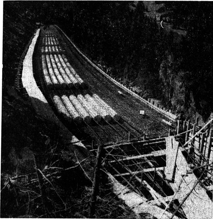
Le ferrailage du pont du Troulero.
