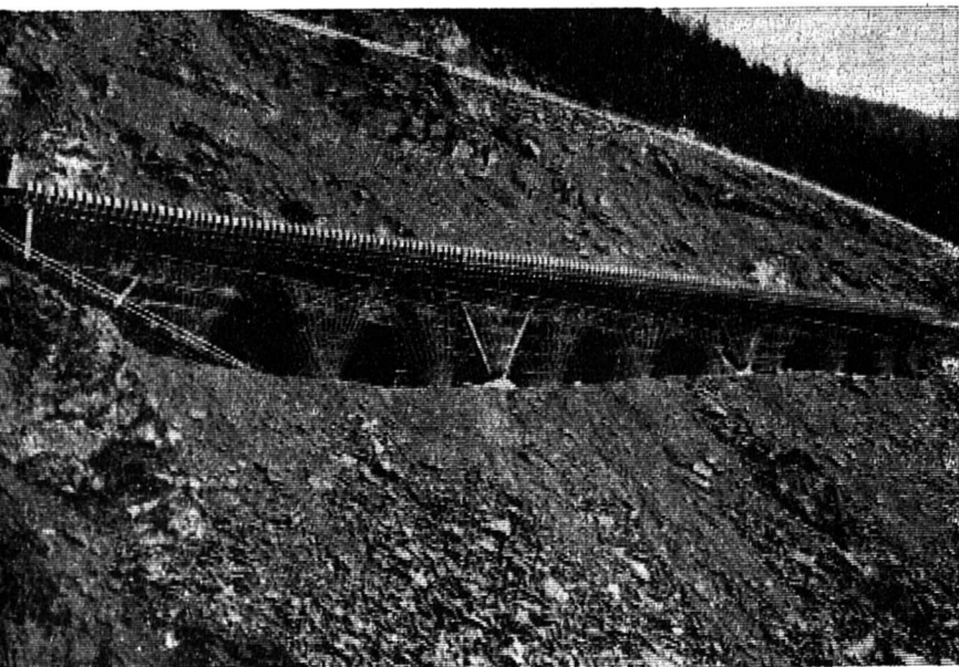
Le même ouvrage vu de la rive gauche de l'Eau-Noire. On remarque les trois points d'appui intermédiaires et l'éboulis en équilibre instable.
