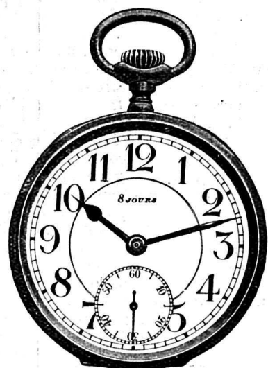
19" Octava, ancre, spiral Breguet, levée visible, 15 rubis, balancier compensé. Or — Argent — Acier — Métal
