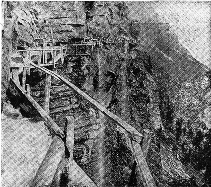
Bisse suspendu, avec passerelle et chéneau, pour gros débit. Le bisse du Torrent-Neuf, à Savièse, accroché depuis le 16e siècle à la paroi des Brantires. (Photos : Paris-Burgat, Lausanne)
