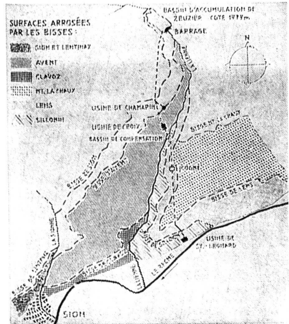
Plan de situation de l'aménagement hydro-électrique de la Lienne et des bissez de la région.
