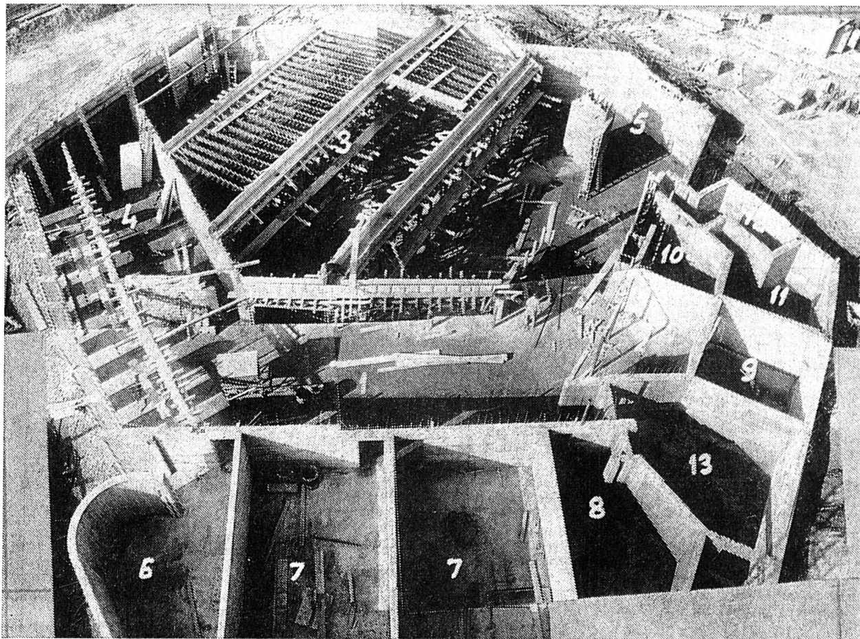
SION — La construction de l'église de St-Guérin progresse. Notre cliché montre une vue d'ensemble des locaux paroissiaux qui sont aménagés sous l'église proprement dite. 1. Entrée et hall; 2. Vestiaires; 3. Salle paroissiale d'une contenance de 300 places; 4. Salle de répétition des chœurs; 5. Cuisine-office; 6. Eclairage; 7. Action catholique; 8. Bibliothèque; 9. Toiletttes et lavabos; 10. Chauffage; 11. Abri P.A.; 12. Cage d'escalier. De plus, une morgue à l'usage de la commune est aménagée en 13.
