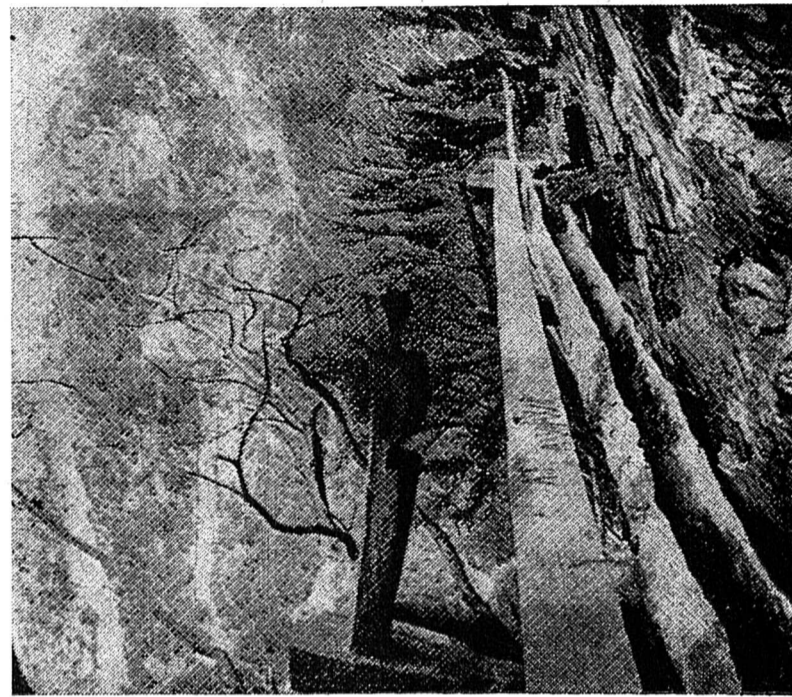
Le bisse de Neuwerk, long de 14 km, dans le Baltschiederthal. Il emprunte ici une étroite corniche. Le rocher en surplomb ne permettant pas de passer sur la banquette du bisse, on a construit une passerelle rudimentaire pour le garde-bisse, faite d'une simple poutre glissante retenue aux extrémités par des arbustes.
