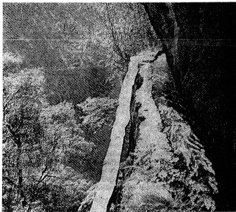
Le bisse «Eggere» dans le Baltschiederthal. Cette conduite d'eau a été construite au 16 e siècle et se compose par endroits de troncs de mélèzes évidés. La passerelle — simple planche posée sur les supports de la conduite — est indispensable pour le passage du garde-bisse au-dessus de l'abîme.
