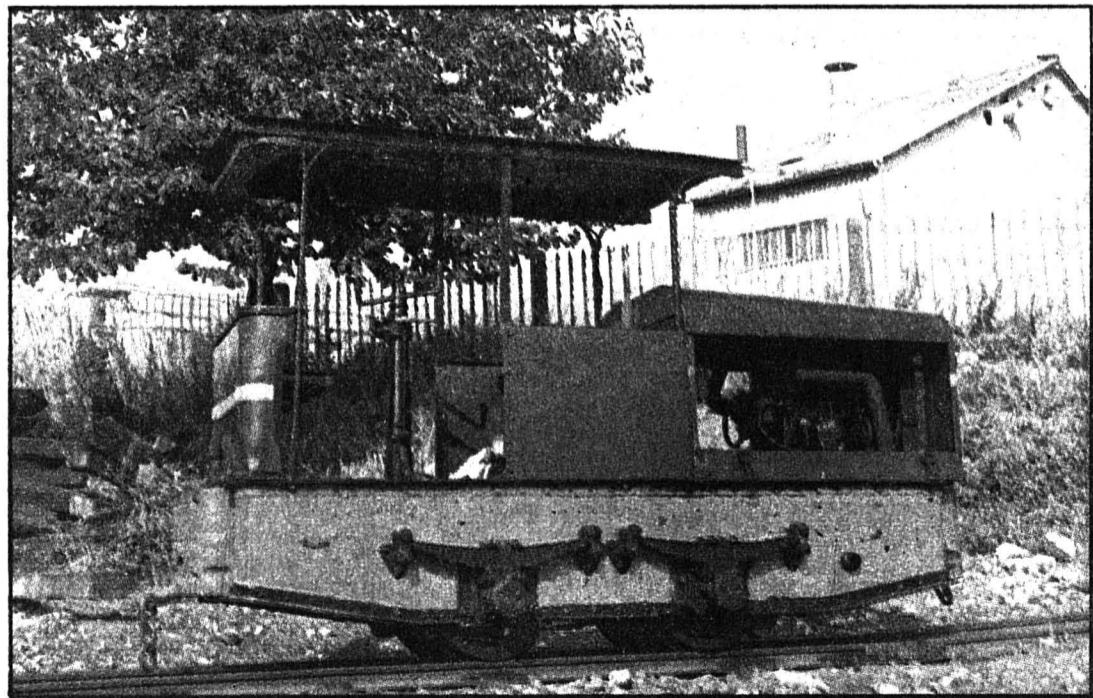
Une des locomotives à essence de la collection Pithiviers.
