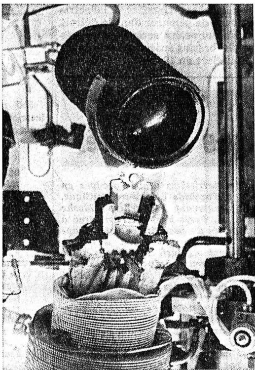
La vitrification des déchets hautement radioactifs est effectuée, à cause de l'intense radiation, avec des machines commandées à distance.
