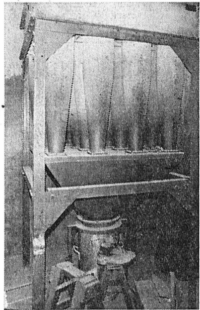
L'installation de dépoussiéreur, très efficace, et qui retient en particulier les suies dont est chargée la fumée.
