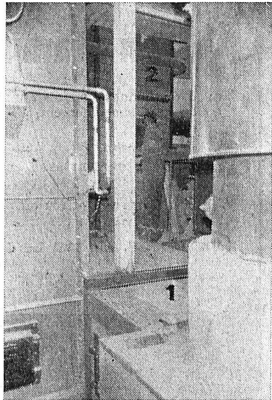
Les cheminées intérieures, en cours de reconstruction. 1. La cheminée horizontale amenant la fumée du four (à droite) au récupérateur de chaleur (à gauche). 2. La cheminée verticale amenant la fumée à l'installation de dépoussiéreur, avant qu'elle ne soit dirigée vers la grande cheminée extérieure.
