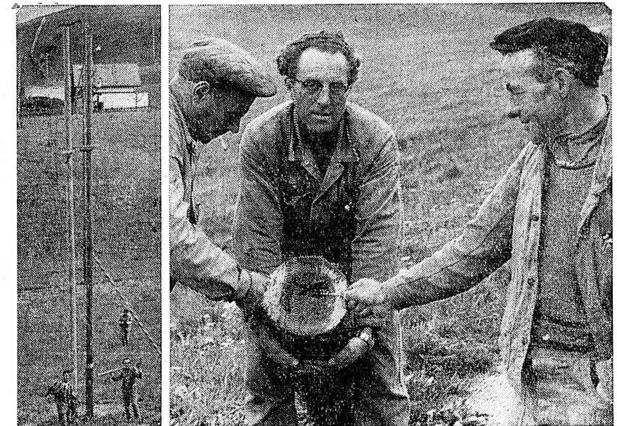
A gauche: La technique employée pour remplacer un poteau ne manque pas d'originalité. Le «malade» est scié à sa base et incliné pour permettre de dresser un nouveau bien portant à sa place. On les fixe alors l'un à l'autre au moyen d'un croisillon de bois jusqu'à l'installation définitive. A droite: On distingue nettement, au centre du poteau, la partie pourrie. Il faut le remplacer avant qu'il y ait danger. (Photos Impartial)
