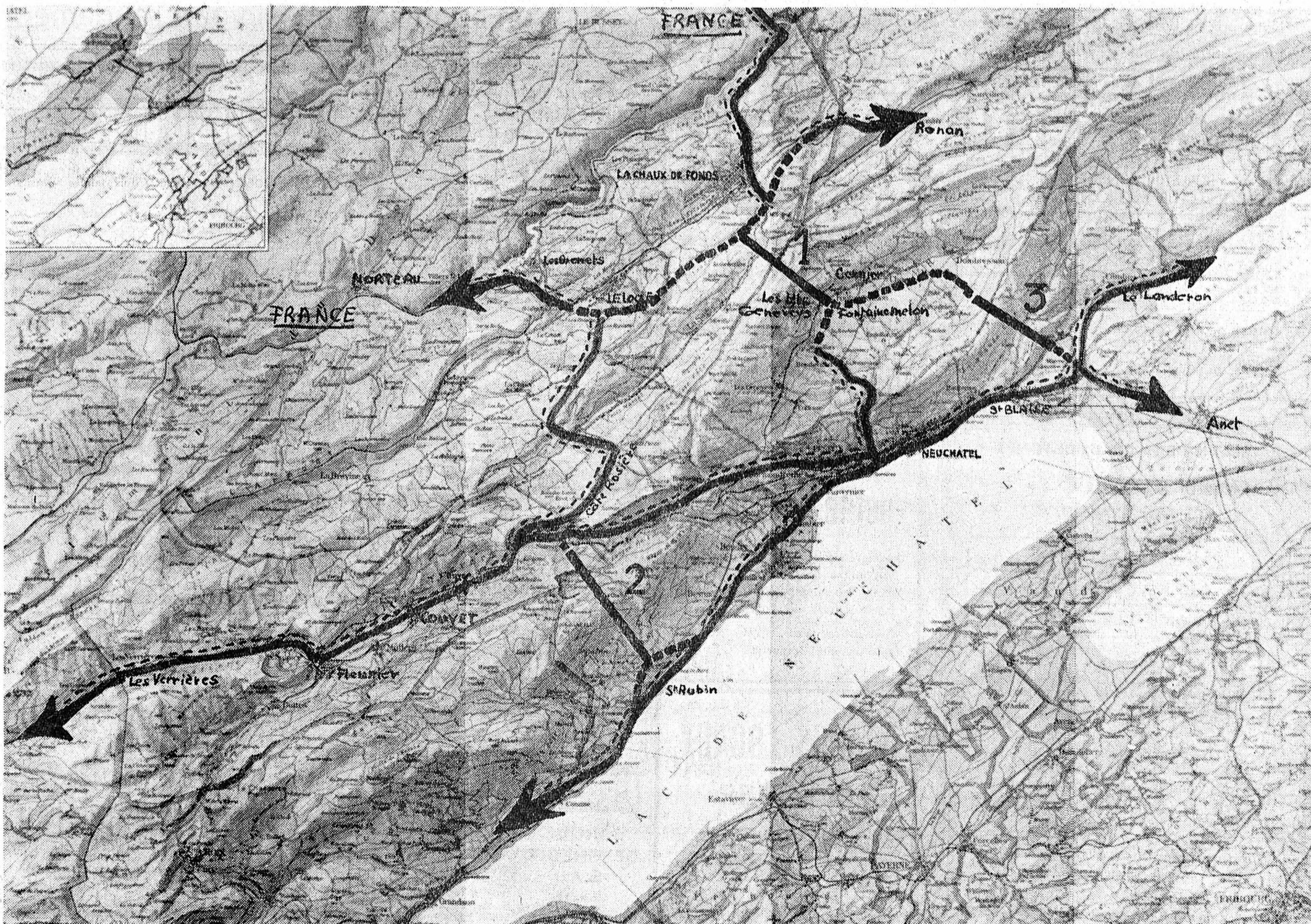
LA POSITION DES TROIS TUNNELS, EN TRAITS PLEINS ET NUMÉROTÉS, 1, 2 ET 3, TELLE QU'ELLE POURRAIT SE PRÉSENTER. LES AUTRES VOIES (EXISTANTES, SOULIGNÉES D'UN POINTILLE), ET CELLES QUI DEVRAIENT ÊTRE CRÉÉES, (EN POINTILLE), N'ONT ICI QU'UNE VALEUR INDICATIVE.
