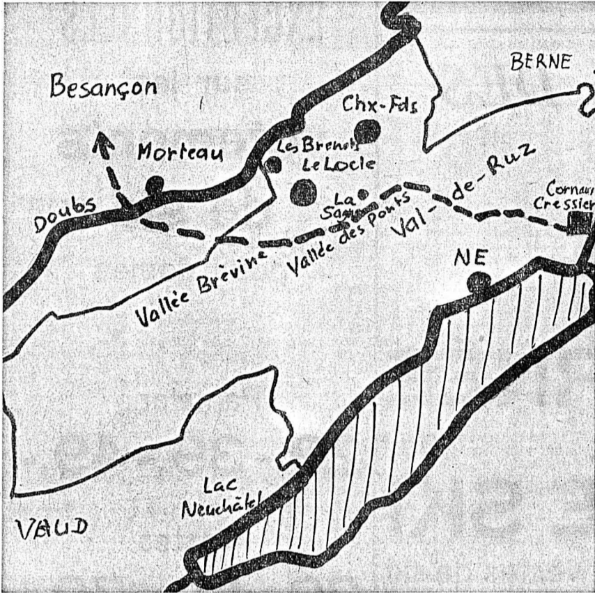
Le tracé approximatif du projet d'oléoduc du Jura : Besançon - Le Gardot - Le Cerneux-Péquignot - La Chaux-du-Milieu - Grand-Sommartel - La Sagne - La Corbatière - La Vue-des-Alpes, Val-de-Ruz - Chaumont - Cressier.
