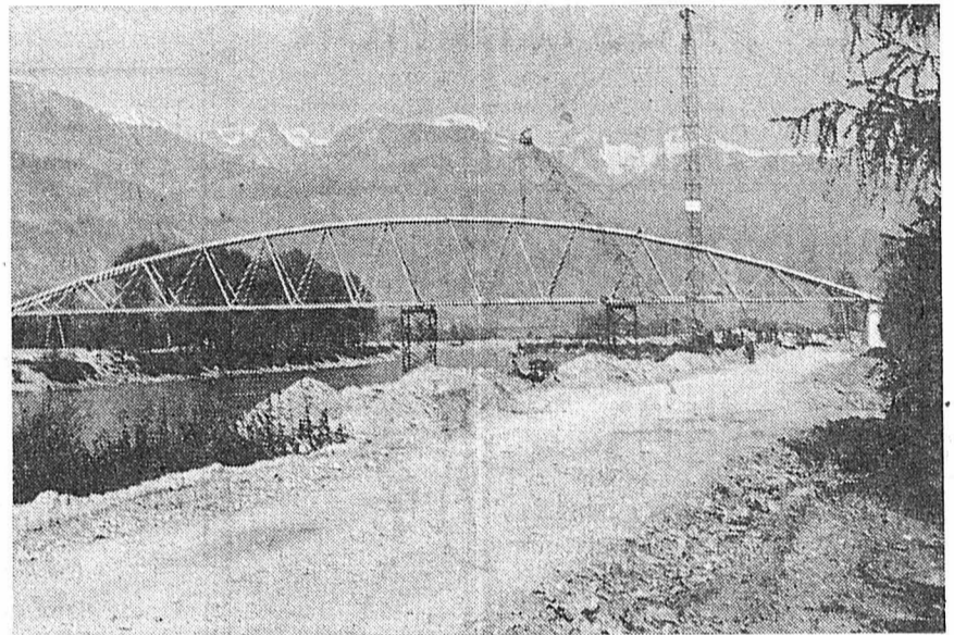
Le pont pipe-line d'Aigle en voie de finition. (Press-Photo-Actualité)
