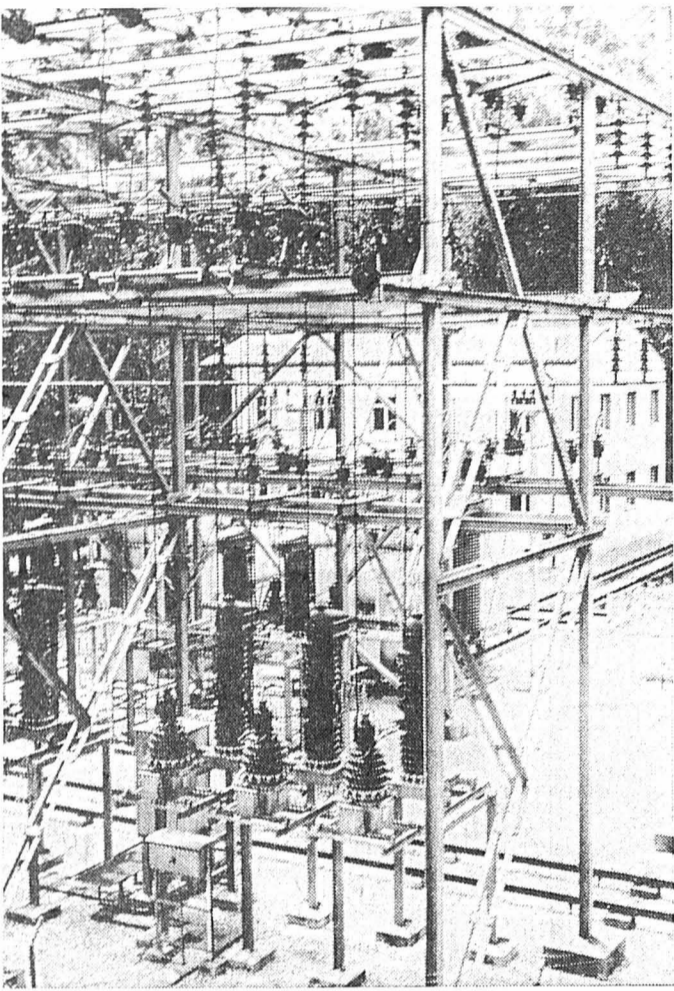
La sous-station de Moutier, alimentée par du courant de 50 000 volts, et d'où rayonnent nombre de lignes de 16 000 volts vers les stations de transformation (Photo Lachat-Mouillet)
