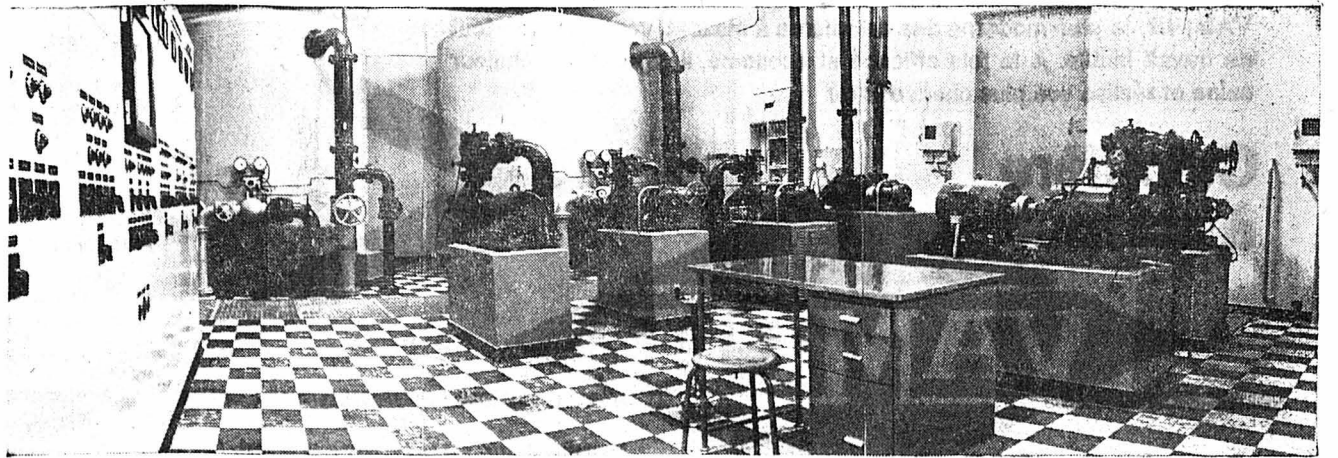
La station de pompage des eaux de la Ronde, qui ravitaille une partie de la ville de La Chaux-de-Fonds. Cette station, qui dispose d'un système d'épuration, est l'une des plus modernes de Suisse.
