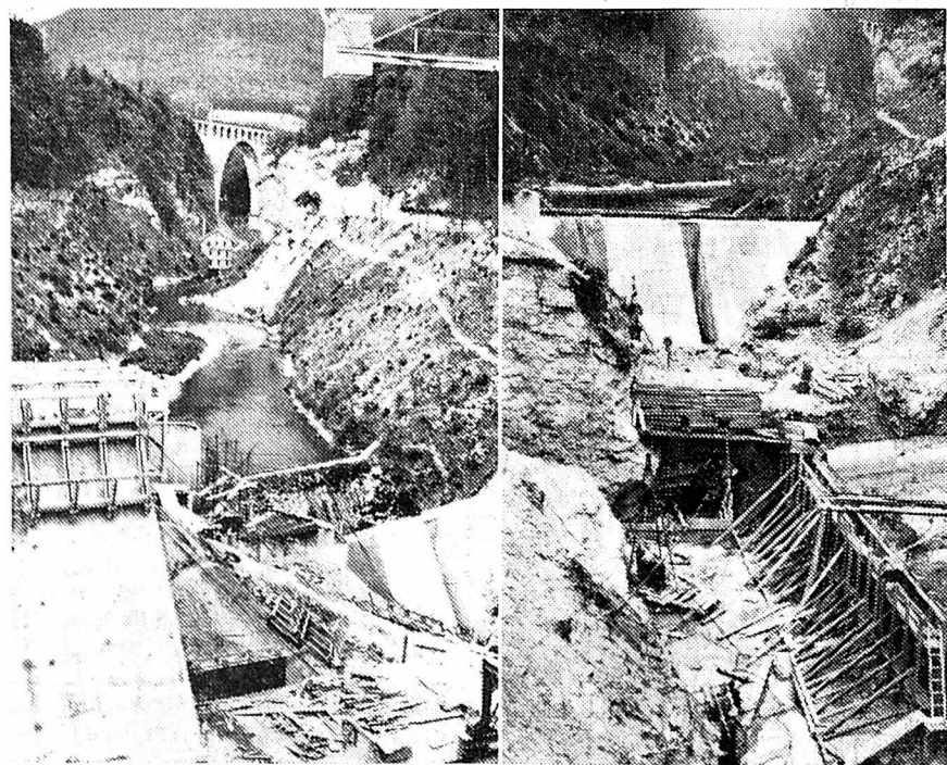
La «Compagnie vaudoise des forces motrices du lac de Joux et de l'Orbe» est en train de construire un nouveau barrage sur le cours de l'Orbe, entre Ballaigues et Moncherand, dont la production annuelle d'énergie sera de 93 millions kwh. Nos photos ont été prises sur le chantier des Clées. La digue du barrage qui s'y élève aura une hauteur de 30 m. et une longueur de couronnement de 90 m. A gauche, on reconnaît au fond le viaduc du Day.
