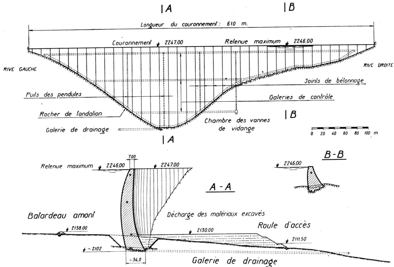
Fig. 4. — Barrage de Moiry. Elévation développée du parement amont, et coupes verticales 1 : 4000
