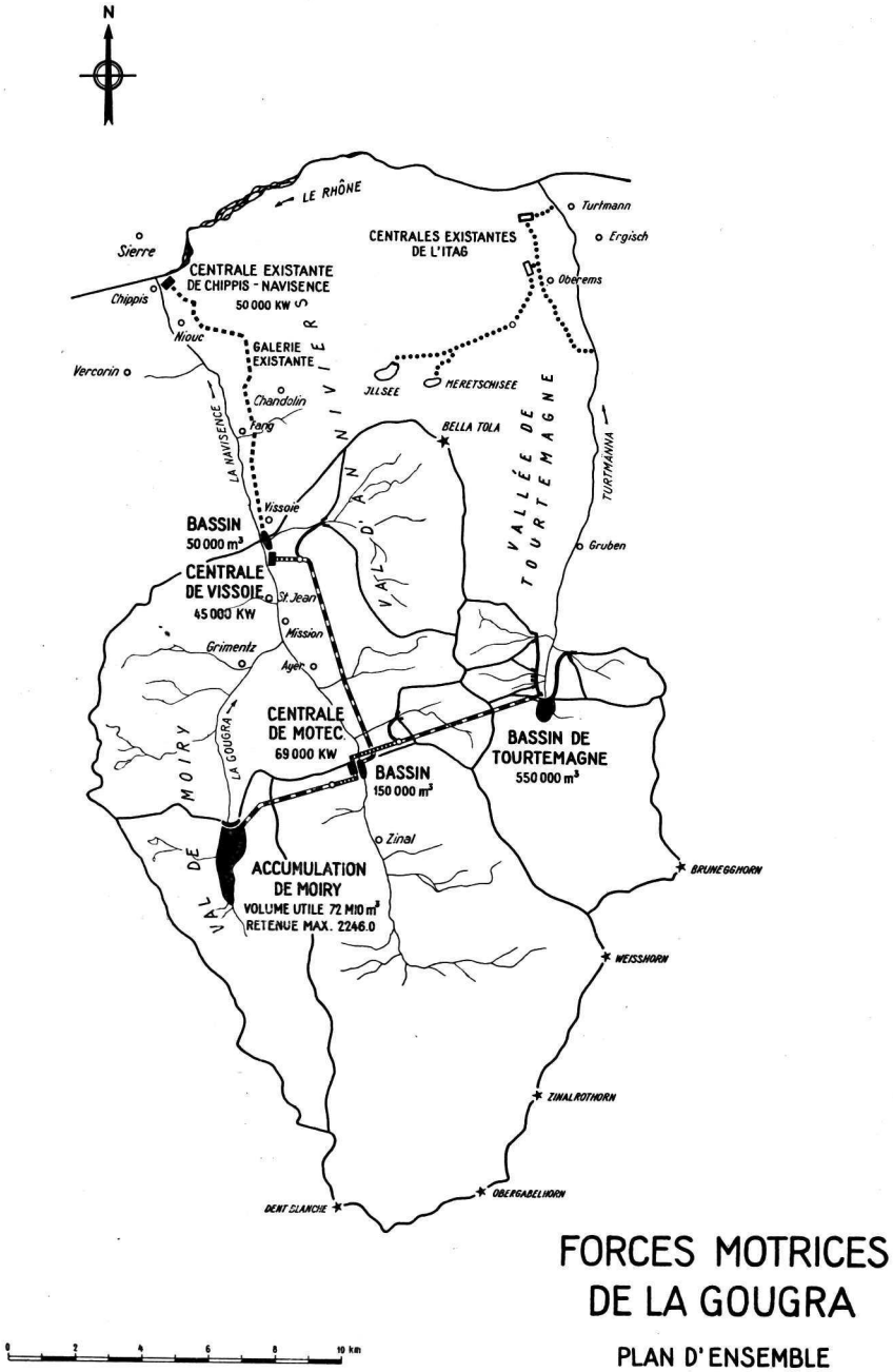
Fig. 1. — Forces motrices de la Gogra. Plan d'ensemble 1 : 300 000
